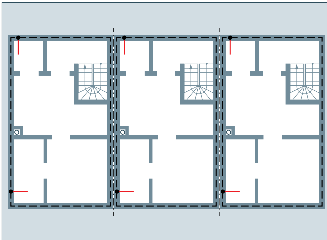
Kuva 3: Perustusmaadoituselektrodi rivitaloissa
