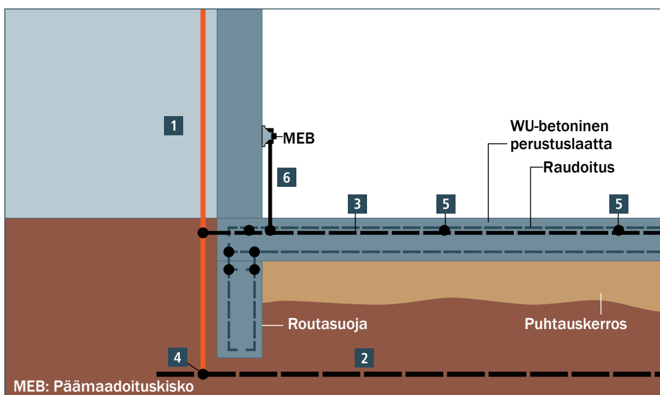
Kuva 6: Toteutus esimerkki, kun on raudoitettu pohjalaatta ja WU-betoninen yhtenäinen raudoitettu perustus
