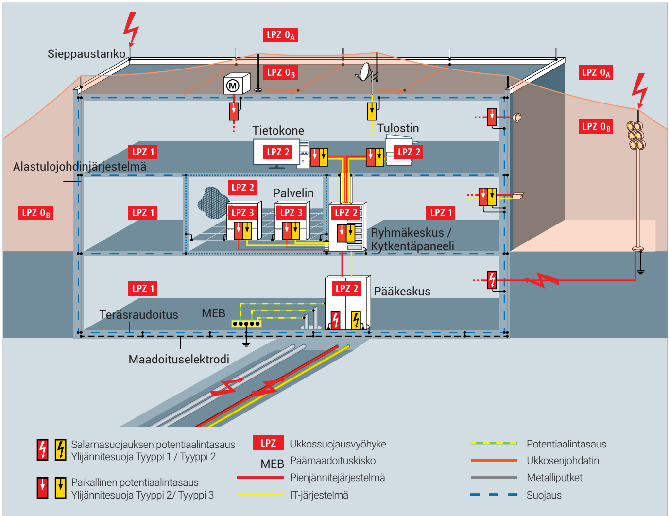
Kuva 1: Yleiskuva ukkossuojaukskonseptista.
