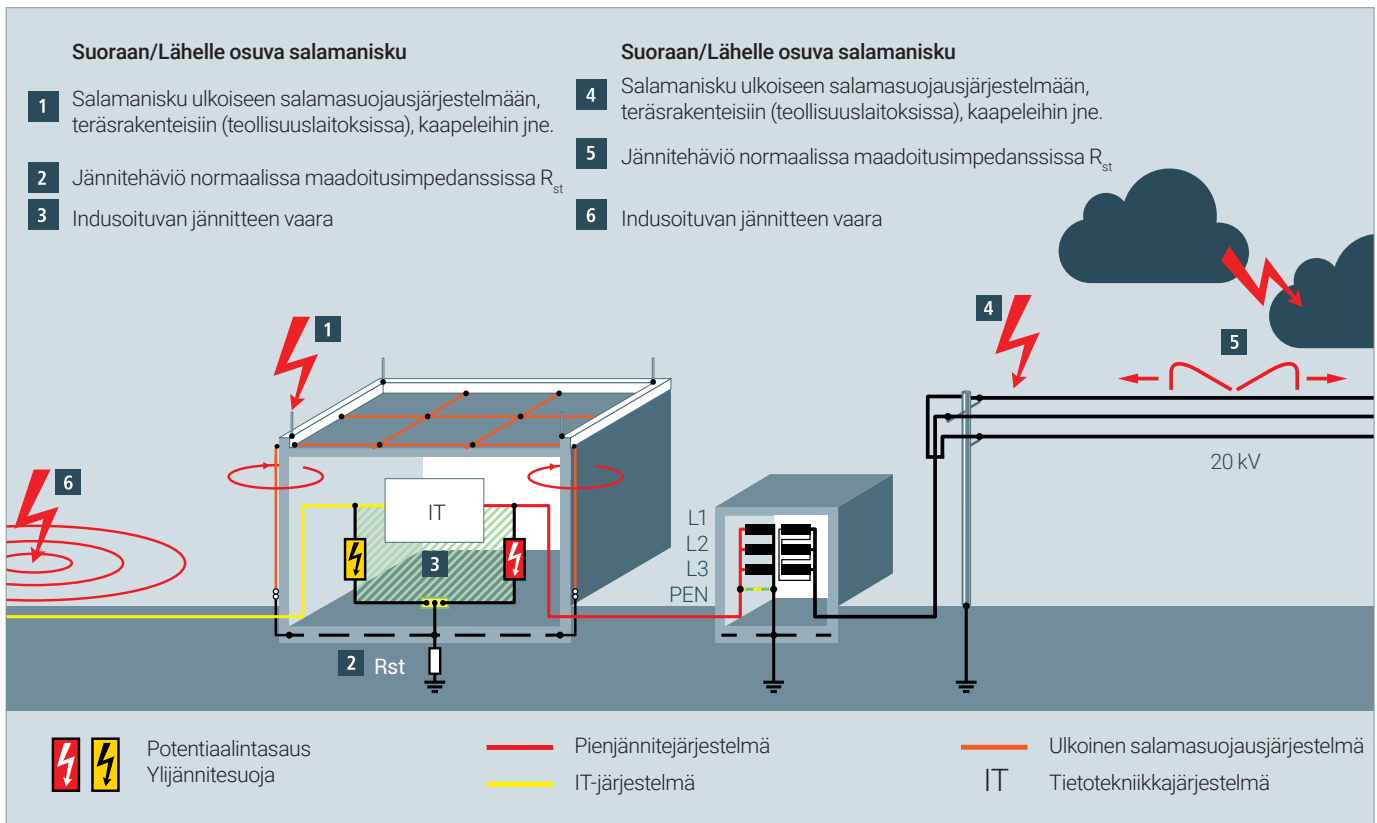
Kuva 2: Salamaniskujen aiheuttamien ylijänniteiden syyt.
