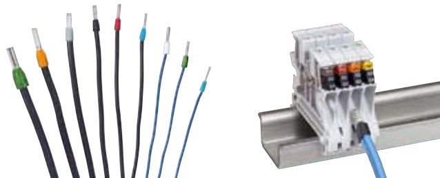
Erlaisia johtoja ja pääteholkkeja
